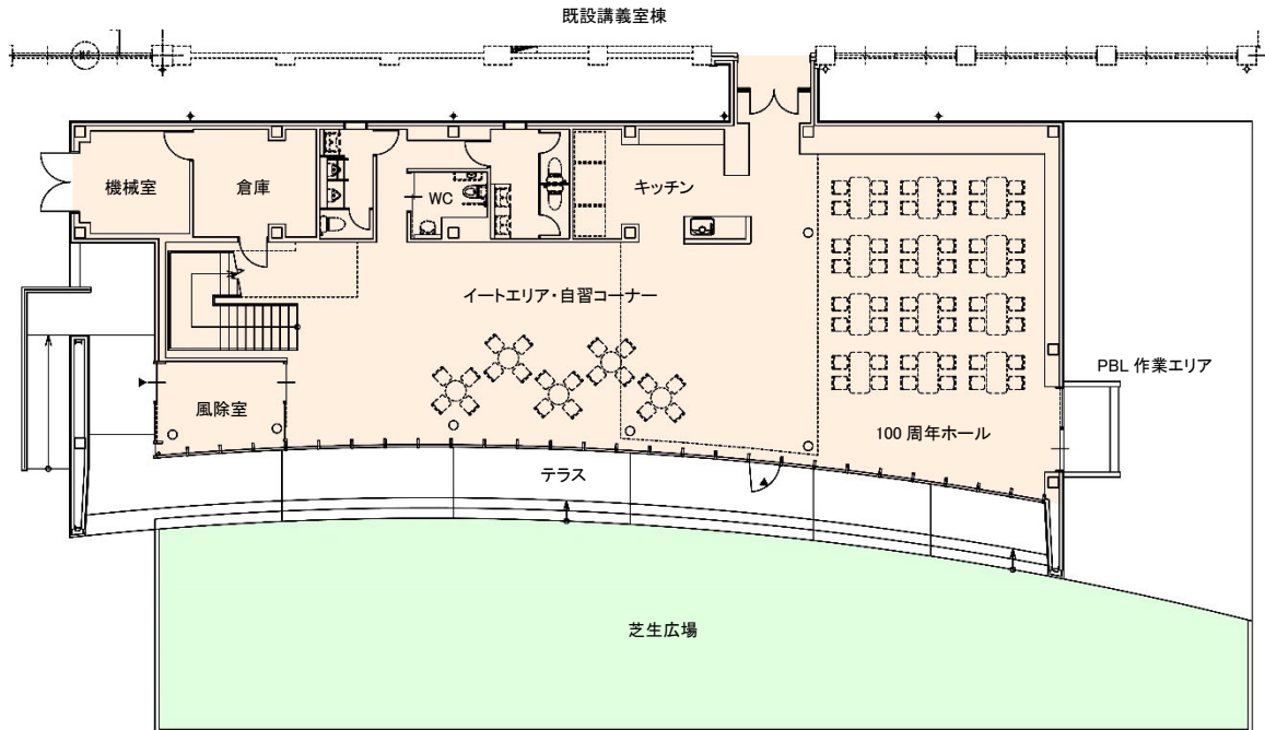
●1階平面図
